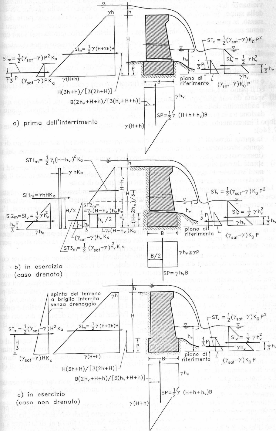
7.14: spinte agenti su una briglia: a: prima dell'interrimento; b: in esercizio (caso drenato); c: in esercizio (caso non drenato).
